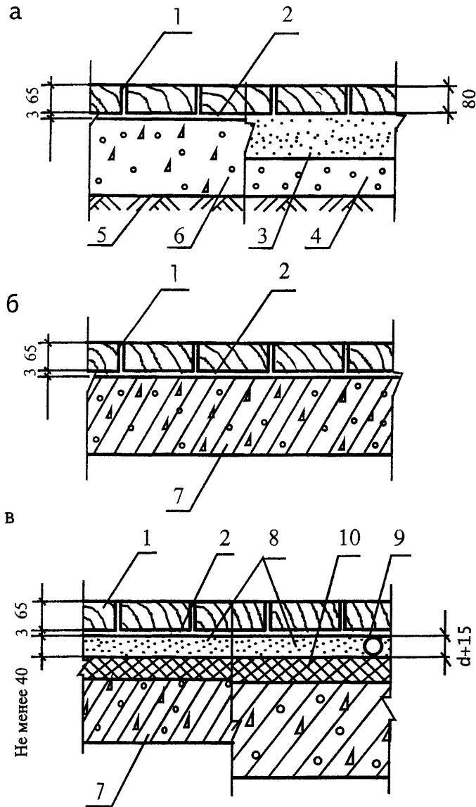
Рис. 17 Конструктивные схемы полов с покрытием из торцевой шашки по подстилающему слою (а) и перекрытию (б)
