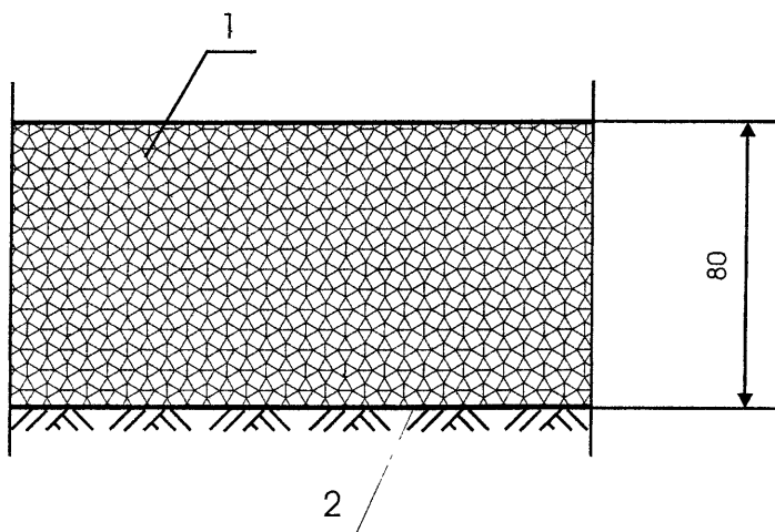
Рис 31 Конструктивная схема полов с глинобитным покрытием 1 – глинобитное покрытие; 2 – грунт основания
