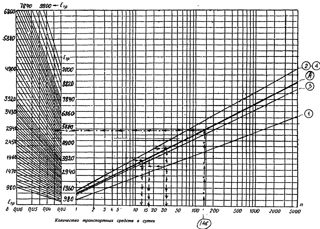
Рис. 4 График для приведения интенсивности движения транспортных средств к интенсивности движения условного автомобиля с расчетной нагрузкой «А» и для определения требуемого модуля деформации E_p пола
