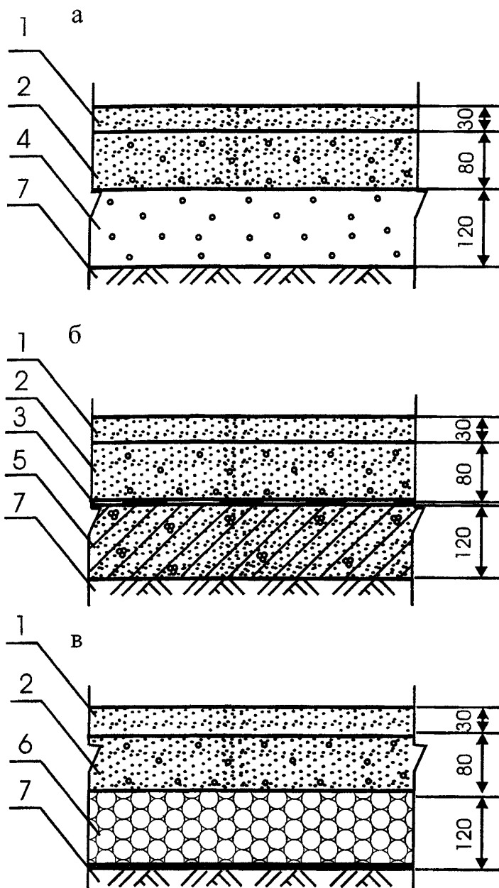
Рис. 12 Конструктивные схемы полов с известняково-керамзитовым покрытием 1 – известняково-керамзитовое покрытие; 2 – теплоизоляционный керамзитовый слой; 3 – гидроизоляция; 4 – подстилающий щебёночный слой; 5 – бетонный подстилающий слой; 6 – подстилающий слой из битумизированного керамзита; 7 – грунт основания
