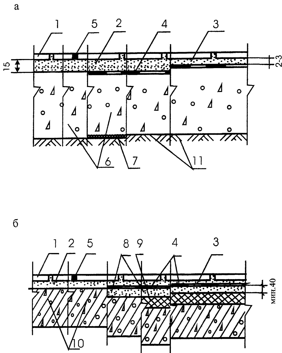
Рис 30 Конструктивные схемы полов с покрытием из плит каменного литья, кислотоупорной плитки и кирпича по подстилающему слою (а) и по перекрытию (б) 1 – плита каменного литья, кислотоупорная плитка и кирпич; 2 – прослойка из цементно-песчаного раствора или раствора на основе жидкого стекла; 3 – прослойка на основе полимерных материалов; 4 – непроницаемый подслоя; 5 – расшивка швов химически стойкими полимерзамазками; 6 – бетонный подстилающий слой; 7 – гравий, пропитанный битумом; 8 – цементно-песчаная или бетонная стяжка; 9 – тепло-звукоизоляция; 10 – плита перекрытия; 11 – грунт основания.
