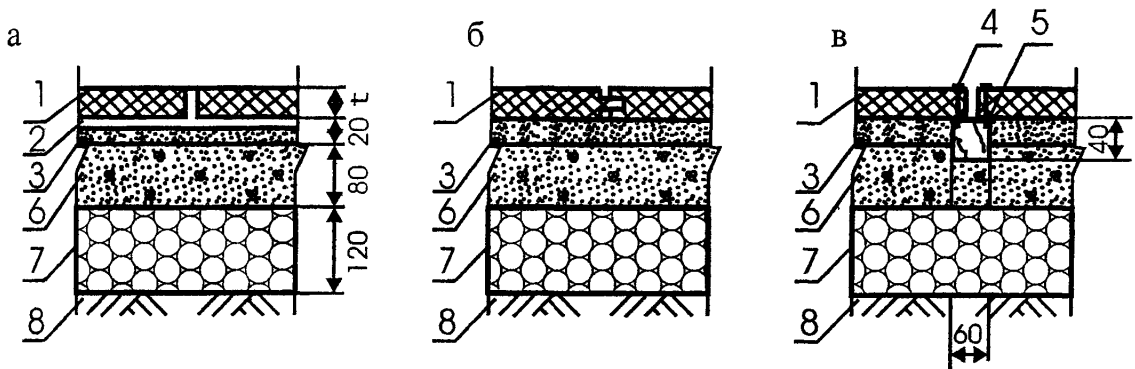
Рис.27 Конструктивные схемы полов в животноводческих зданиях с покрытием из резиновых, резинокордовых и резинокордобитумных плит, уложенных на клеящую прослойку (а), насухо (б) и прикрепляемых к деревянным брускам (в) 1 – плиты резиновые, резинокордовые и резинокордобитумные с ровной нижней поверхностью; 2 – клеящая прослойка; 3 – стяжка; 4 – шиферный гвоздь; 5 – антисептированный деревянный брус 40х60 мм; 6 – теплоизоляционный слой из лёгкого бетона; 7 – подстилающий слой (щебень крупностью 40-60 мм, пропитанный битумом); 8 – грунт основания
