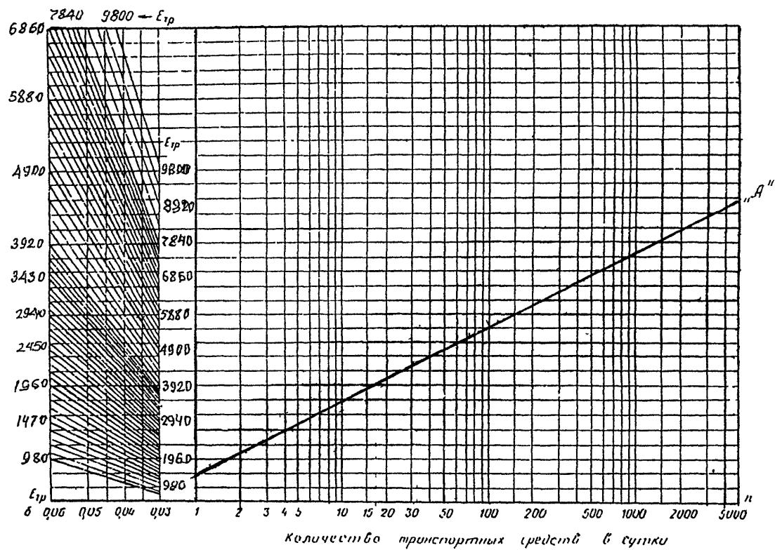
Рис 4 График для приведения интенсивности движения транспортных средств к интенсивности движения условного автомобиля с расчетной нагрузкой «А» и для определения требуемого модуля деформации E_{тр} пола
