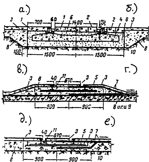
Рис. 6 Полы в зоне железнодорожных путей а). колеи 1524 мм с покрытием из железобетонных плит;
