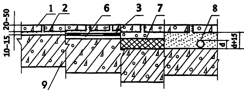
Рис 6 Конструктивные схемы полов с покрытием из бетонных и мозаичных плит по подстилающему слою (а) и по перекрытию (б) 1 – плиты покрытия; 2 – прослойка; 3 – гидроизоляция; 4 – бетонный подстилающий слой; 5 – грунт основания; 6 – стяжка; 7 – тепло-звукоизоляция; 8 – трубопровод; 9 – плита перекрытия.
