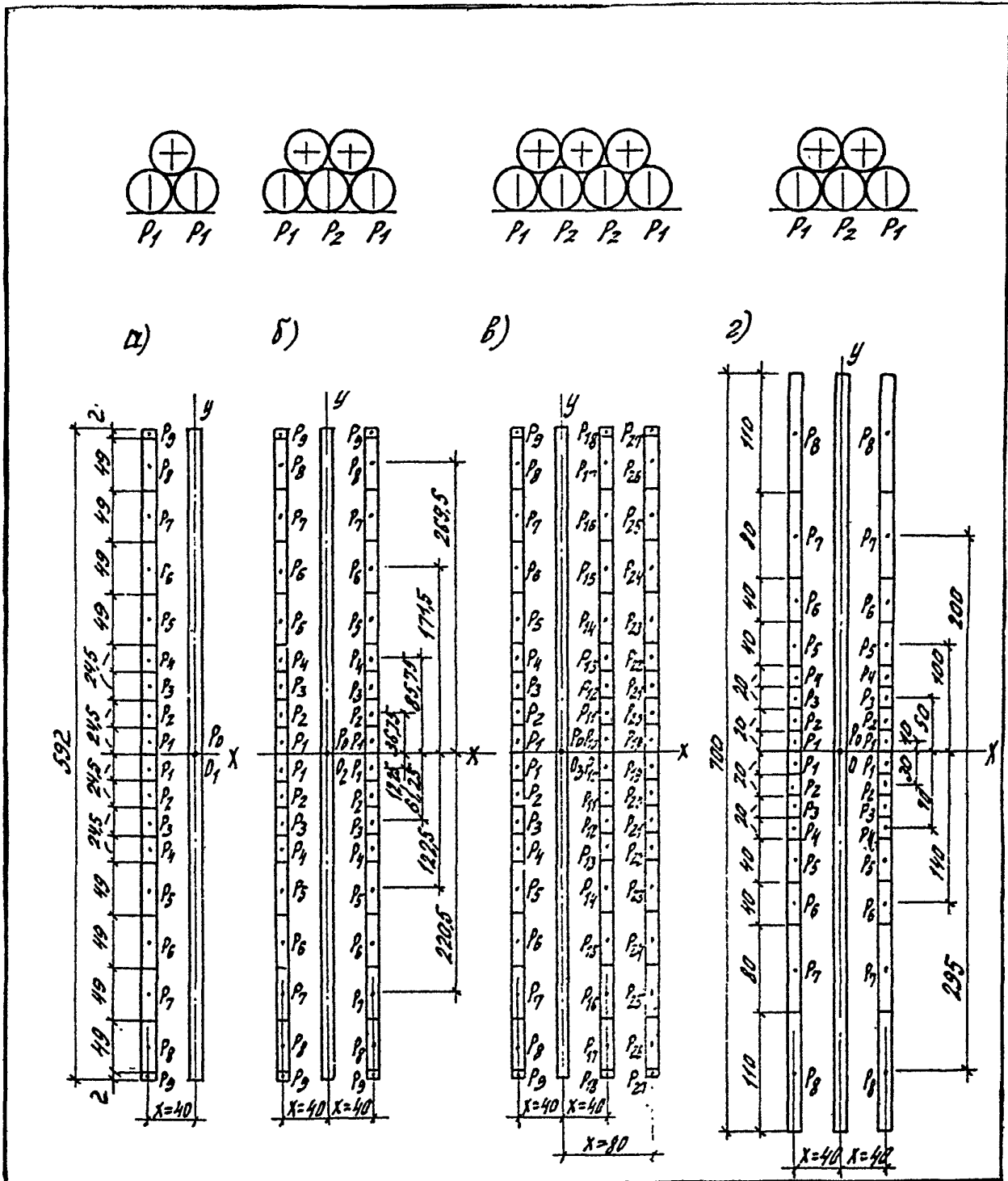
Рис. 3 Схема расположения в плане нагрузок от валов, расчётных центров O , осей координат и разделения следов нагрузок на элементарные площадки
