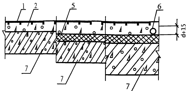
Рис. 15 Конструктивные схемы полов с покрытием из чугунных и стальных плит по подстилающему слою (а) и перекрытию (б)
