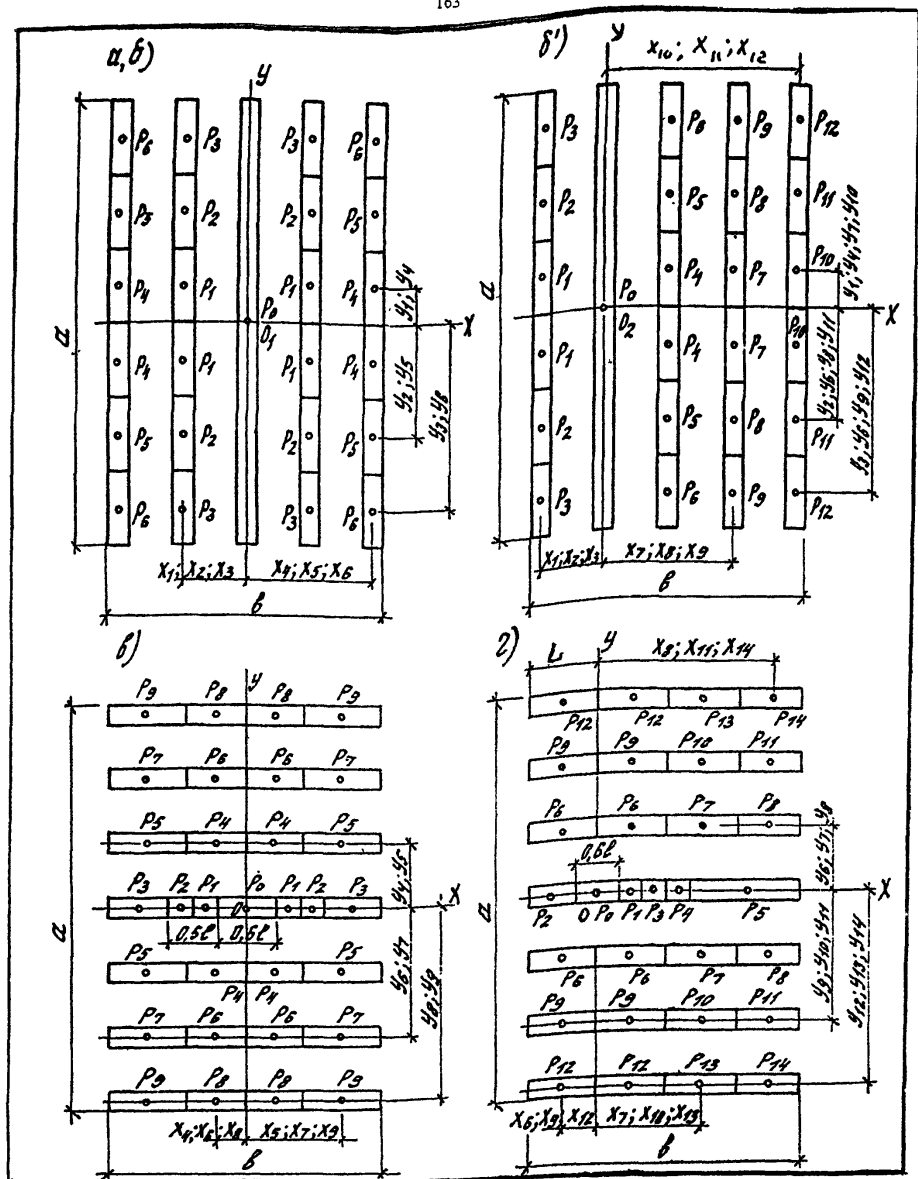
Рис. 2 Схема расположения в плане нагрузок сложного вида, расчётного центра O , осей координат и деления следов нагрузок на элементарные площадки а, в – нагрузки, равномерно распределённые по длине параллельных следов (от прокладок под тяжёлые предметы, от штабелей цилиндрических валов и др.) при b \leq 4,4 \cdot l ; a > b ; б; г – то же при b > 4,4 \cdot l ; a > b
