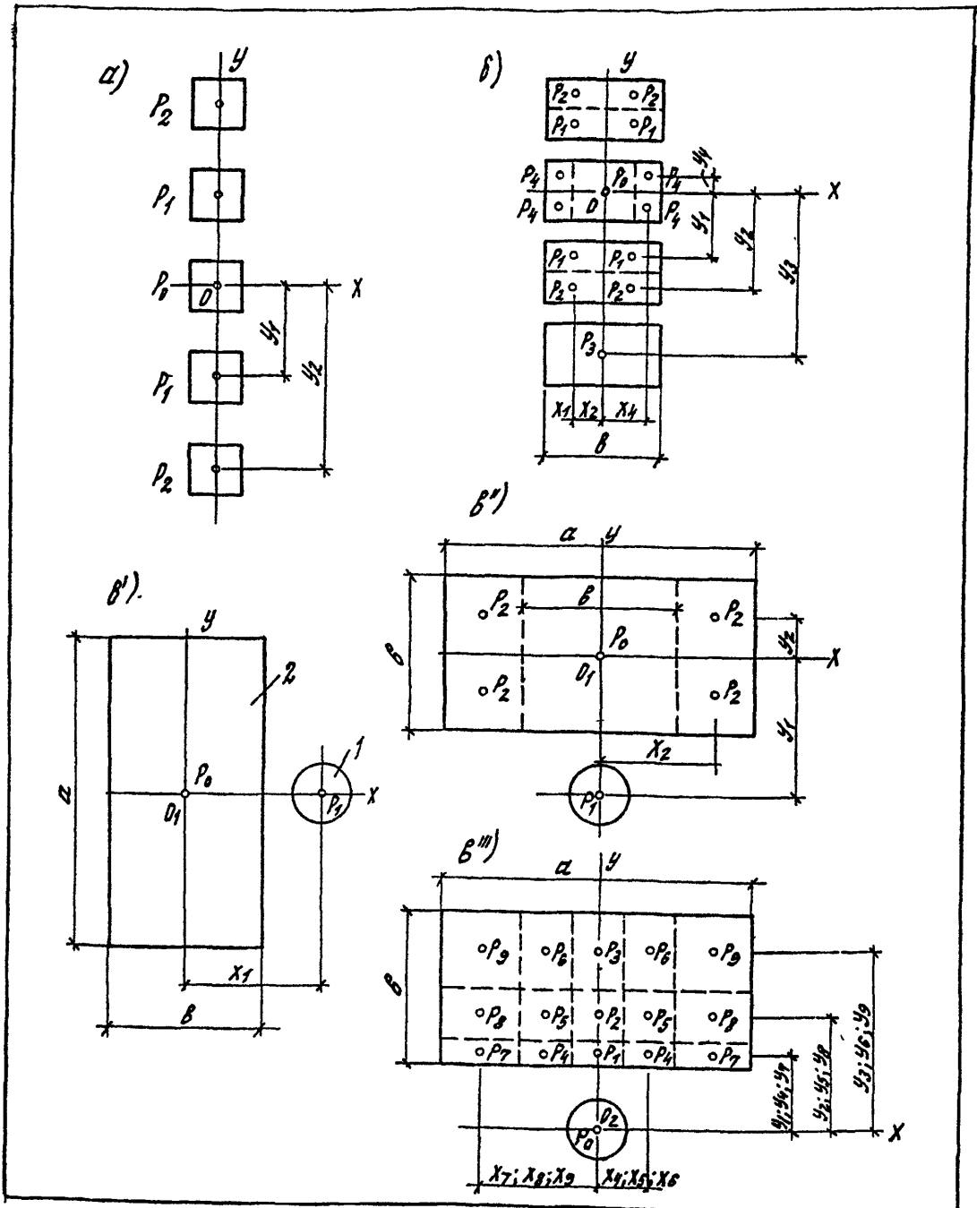
Рис. 1 Схема расположения в плане нагрузок сложного вида, расчётного центра O , осей координат и разделения следов нагрузок на элементарные площадки а – нечётное количество одинаковых нагрузок, расположенных в один ряд; б – то же при четном количестве нагрузок b \leq 4,4 \cdot l ; в (в'; в''); в''') – нагрузка разной величины с различными площадями следов; 1 – след колеса транспортного средства, след станка, агрегата
