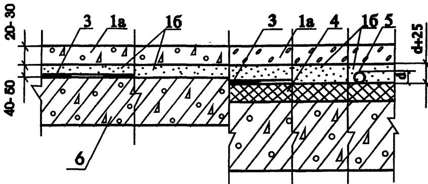
Рис 5 Конструктивные схемы полов с мозаично-бетонным покрытием по подстилающему слою (а) и по перекрытию (б)
