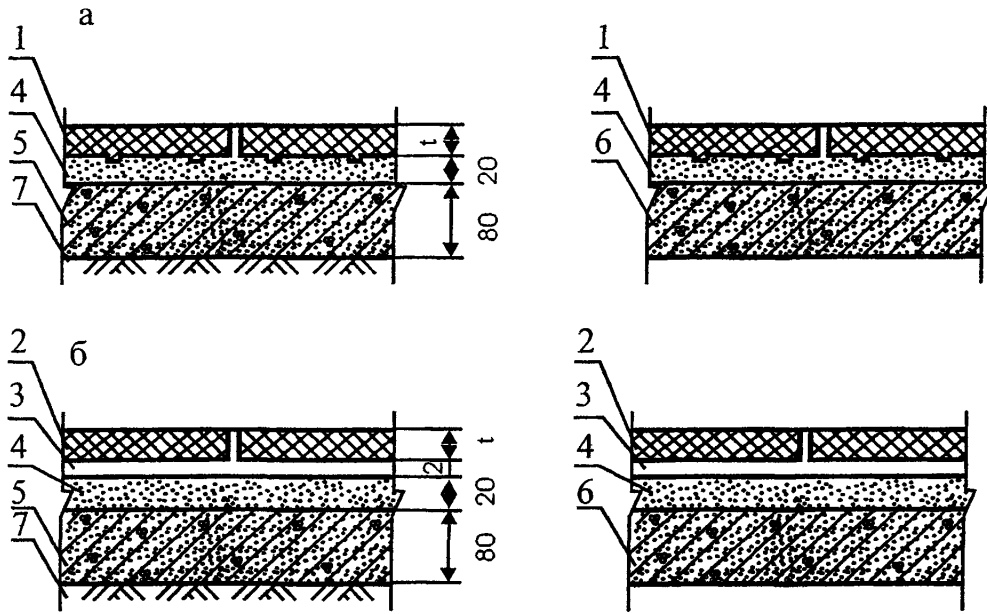
Рис.26 Конструктивные схемы полов в производственных зданиях с покрытием из резиновых, резинокордовых и резинокордобитумных плит, уложенных на свежеприготовленный цементно-песчаный раствор (а) и клеящую прослойку (б) 1 – плиты резиновые с анкерами, 2 – плиты резиновые, резинокордовые и резинокордобитумные с ровной нижней поверхностью; 3 – клеящая прослойка, 4 – стяжка, 5 – бетонный подстилающий слой, 6 – плита перекрытия, 7 – грунт.
