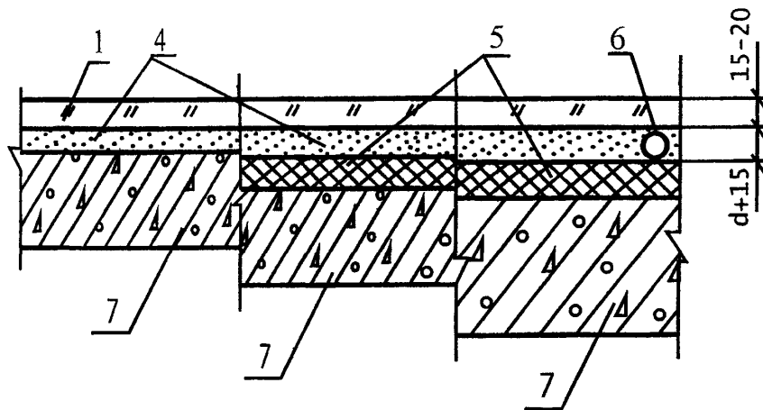
Рис 13 Конструктивные схемы полов с ксилолитовым и поливинилацетатце- ментно-опилочным покрытием по подстилающему слою (а) и пере- крытию (б)
